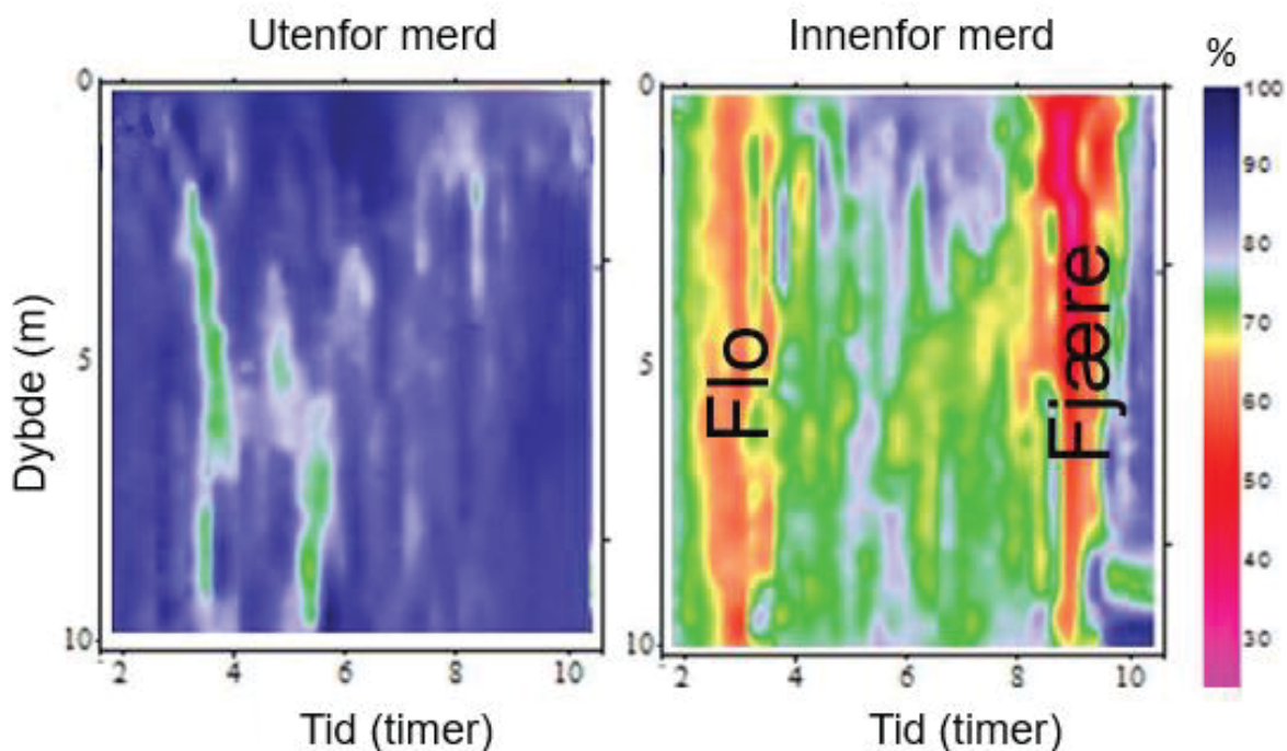
Figur 3.2-2. Eksempel på hypoksiske tilstander inne i en merd i perioden mellom flo og fjære («når den snur») når det er nesten strømsstille. Illustrasjon tilpasset fra [84].
